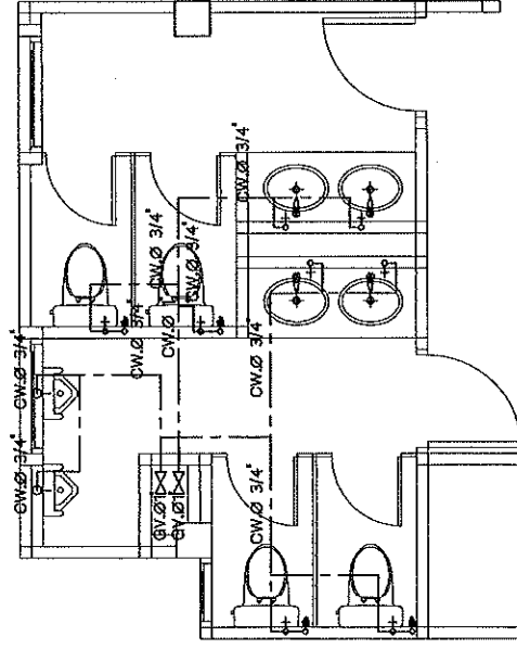
แบบแสดงแนวท่อน้ำดี
