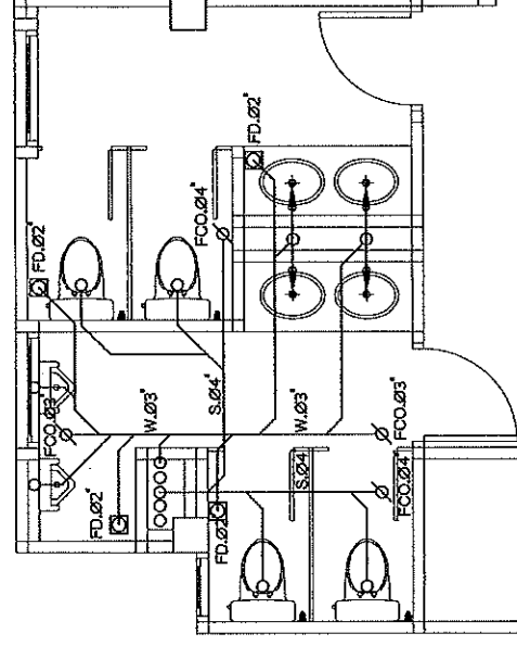
แบบแสดงแนวท่อน้ำทิ้ง
